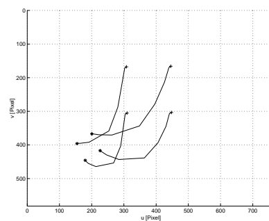
(d) Trust-Region-Regler, d_{soll} = 0.5 mm (8 Schritte)
