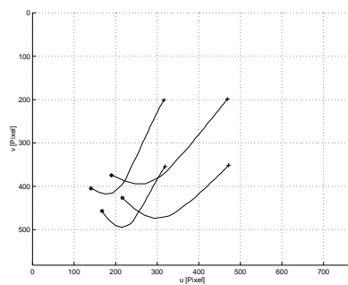
(a) Traditioneller Regler, k = 0.07 (85 Schritte)
