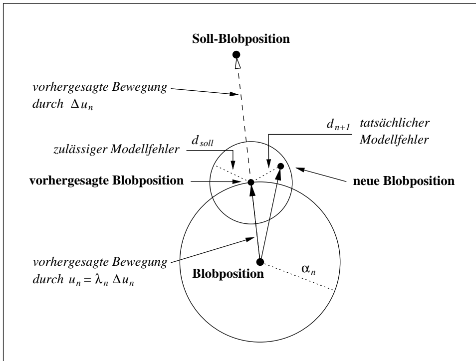
Bild 3: Konstruktion einer Stellgröße mit Hilfe einer bildbasierten Trust-Region-Methode — Betrachtung einer abgebildeten Objektmarkierung (“Blob”) auf dem CCD-Sensor
