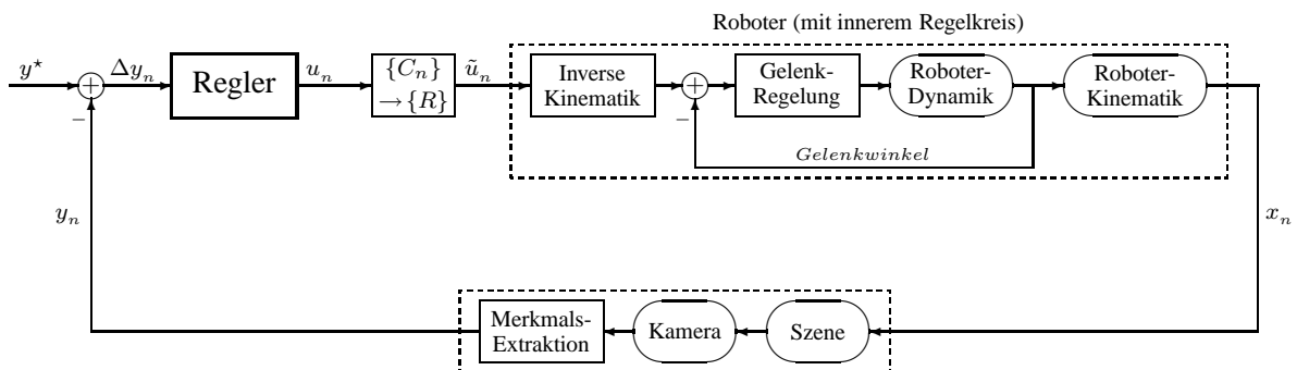
Bild 2: Geschlossener bildbasierter Regelkreis
