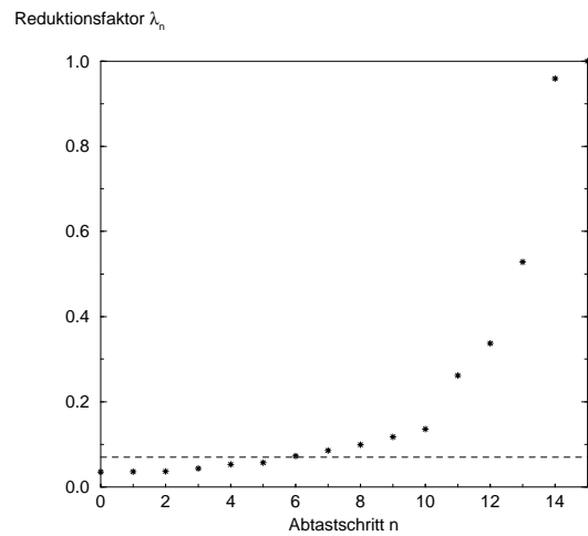
(b) Erfolgte Reduktion der Kamerabewegung
