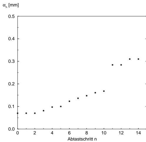
(a) Verlauf der Schranke \alpha_n
