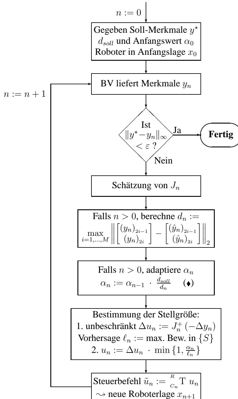
Bild 4: Ablaufplan einer Regelung mit dem Trust-Region-Regler (◆) abhängig von Reglerparametern; siehe Abschnitt 5.3
