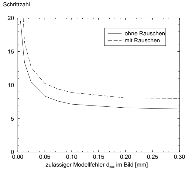
Bild 10: Anzahl Regelschritte bei adaptiver Beschränkung des Schrittes im Bild
