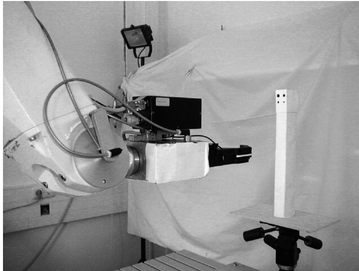
Bild 1: Systemaufbau mit Roboterarm, Kamera und Objekt
