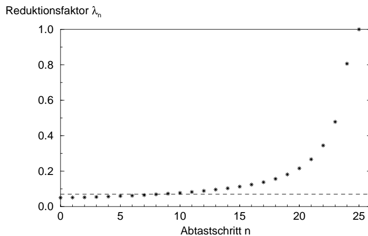
Bild 7: Erfolgte Reduktion der Kamerabewegung (Faktor \lambda_n )
